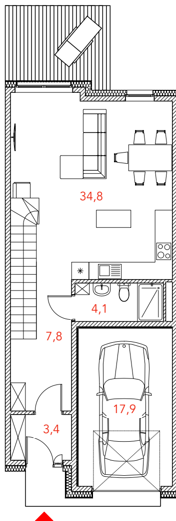
RZUT PARTERU
