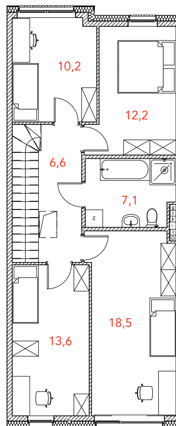
RZUT PIĘTRA
