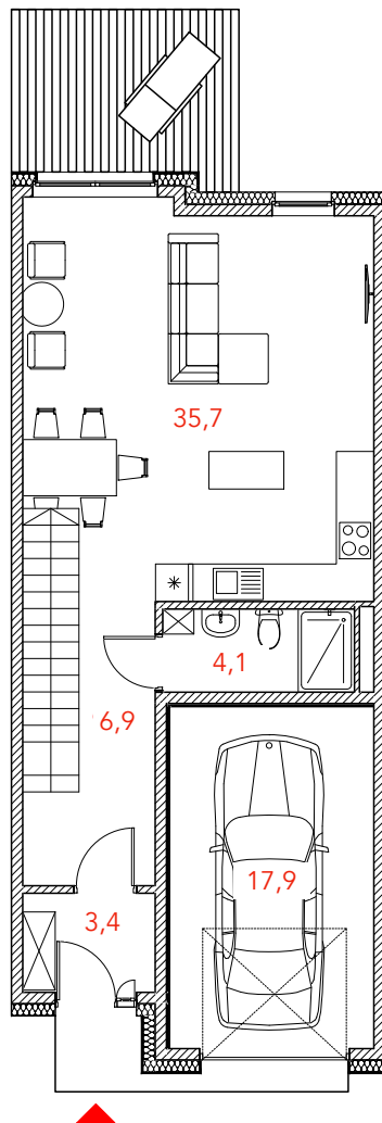
RZUT PARTERU
