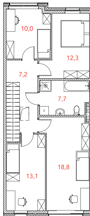
RZUT PIĘTRA
