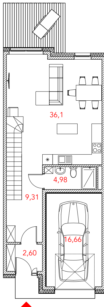
RZUT PARTERU
